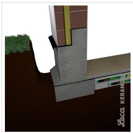
1. Wykop obwodowy wzdłuż ścian fundamentowych
