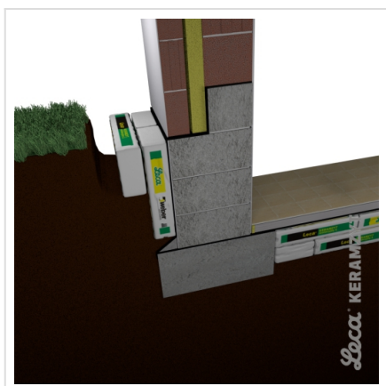
5. Ustawienie drugiej warstwy worków z Leca® KERAMZYTEM izolacyjnym L
