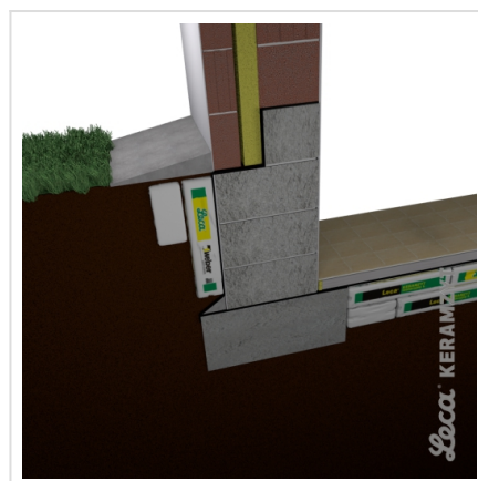
6. Wyrównanie gruntu i ułożenie opaski betonowej
