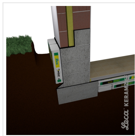
4. Podsypka pod następną warstwę
