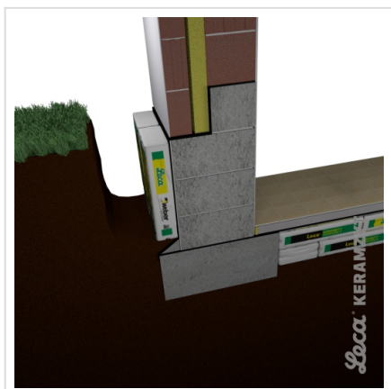
3. Ustawienie worków z Leca® KERAMZYTEM izolacyjnym L
