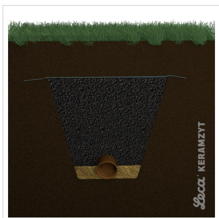
5. Wyrównanie terenu i ew. podbudowa oraz nawierzchnia
