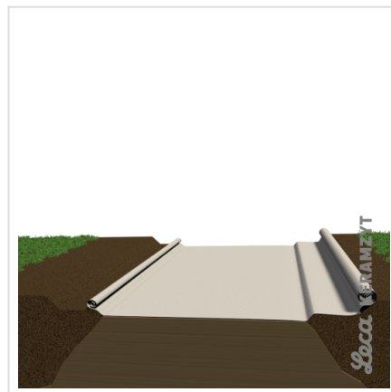
2. Ułożenie geotkaniny na dnie wykopu z zapasami
