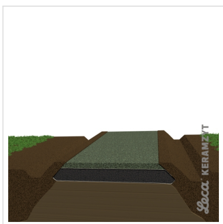
5. Ułożenie podbudowy drogi i poboczy
