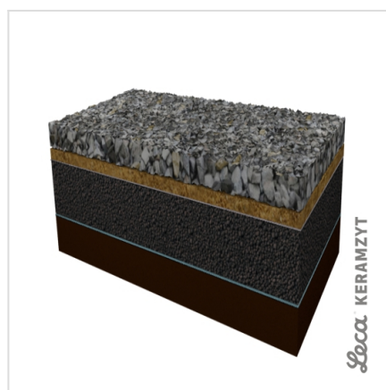
6. Podbudowa z kruszywa kamiennego 31,5-63 mm
