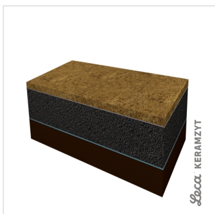
5. Podkład z warstwy piasku
