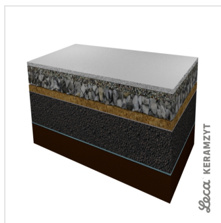
8. Warstwa miążu kamiennego 0-4 mm
