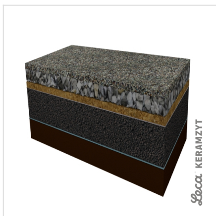
7. Podbudowa z kruszywa kamiennego 0-31,5 mm
