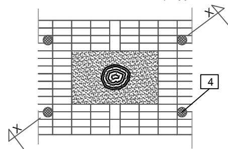
Rozmieszczenie kratki ściekowej [4]
