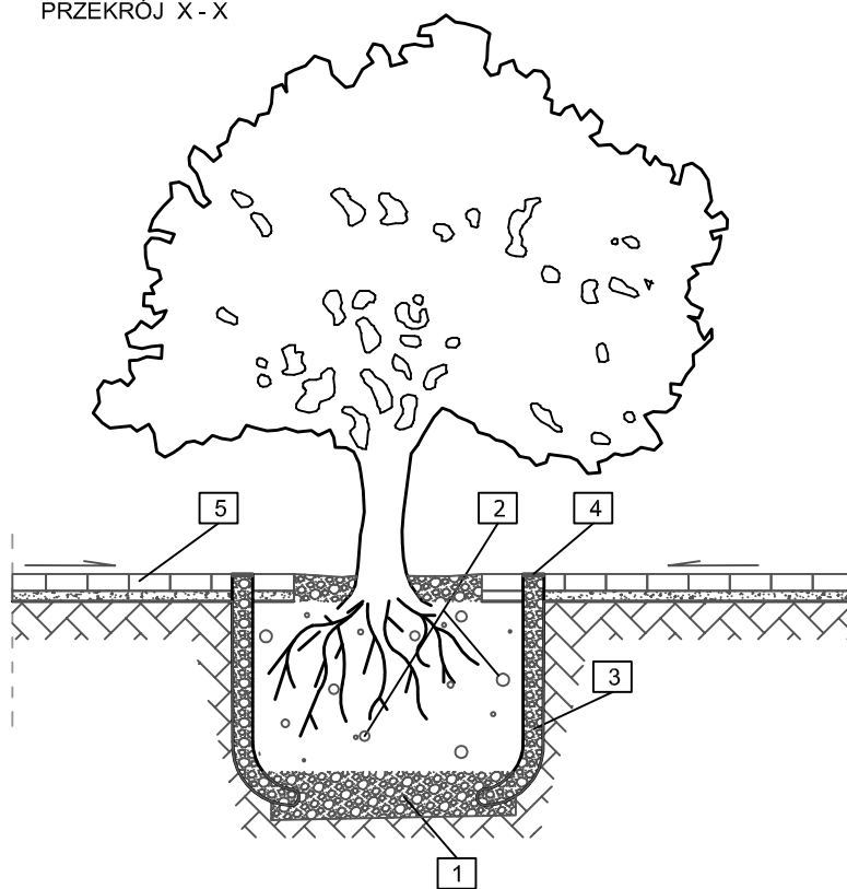
PRZEKRÓJ X - X
