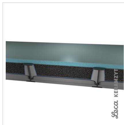
6. Folia odbłaskowa (metalizowana)
