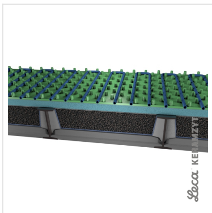
7. Rurki ogrzewania na macie kształtującej ich trasę
